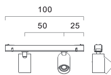
MINITRACK EYES-L2-24V
