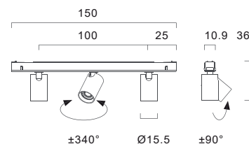
MINITRACK EYES-L3-24V
